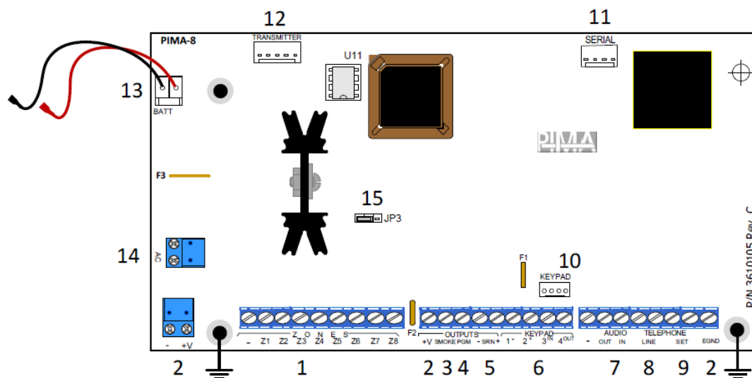
Рисунок 1 - Эскиз платы ППКОП CAPTAIN-I(8)
