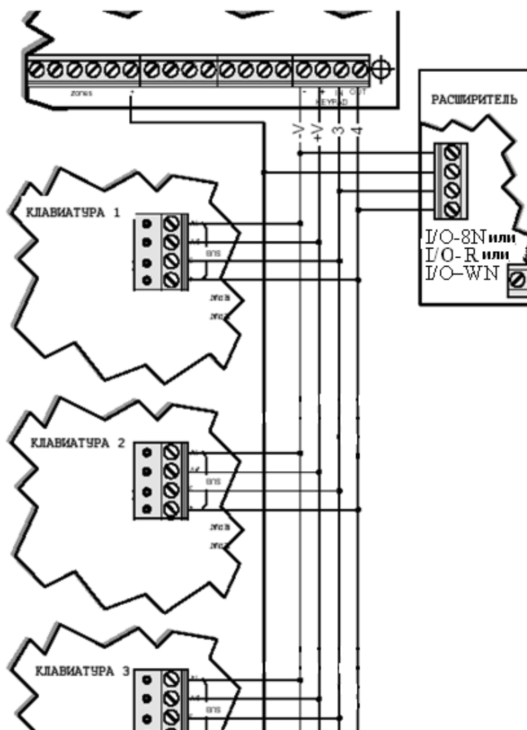
Рисунок 21 - Подключение расширителей и клавиатур без дополнительного источника питания
