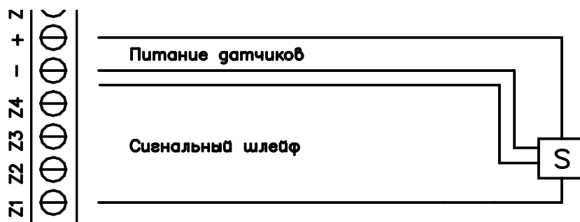
Рисунок 2 - Подключение датчиков к ППКОП CAPTAIN-I(8)
