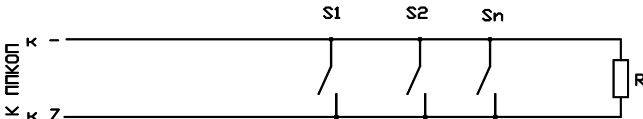
Рисунок 5 - Формирование шлейфов с одним оконечным резистором из нормально разомкнутых датчиков
