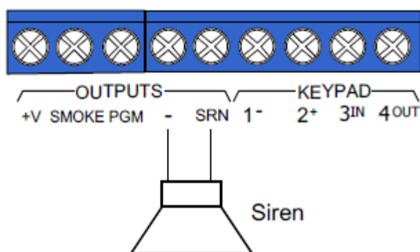
Рисунок 12 - Подключение сирены
