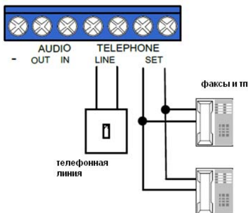
Рисунок 25 - Подключение телефонной линии и дополнительных устройств
