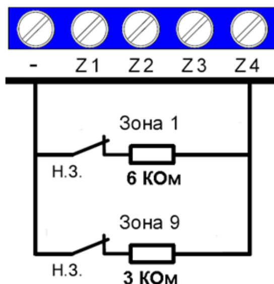
Рисунок 8.1 - Пример формирования шлейфов с использованием функции «Удвоение зон»
