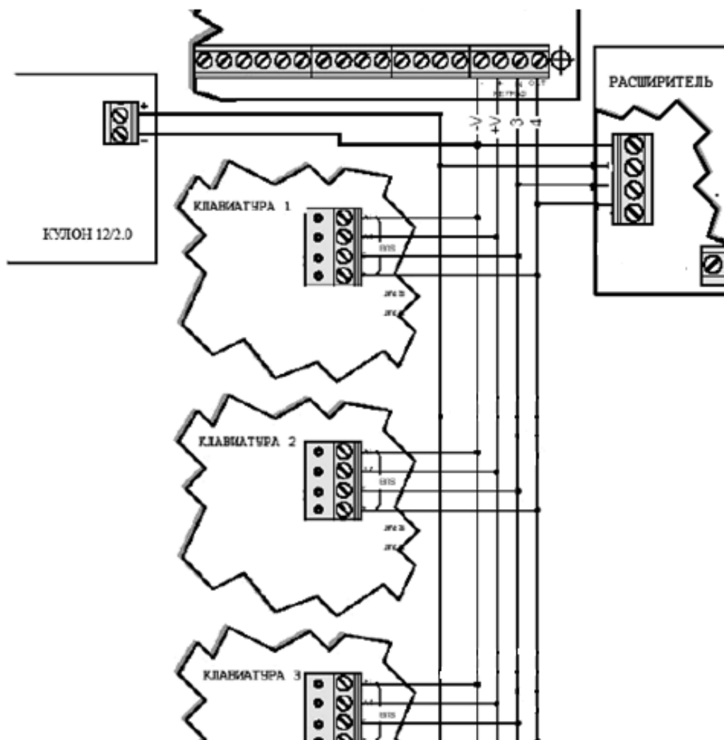
Рисунок 22 - Подключение расширителей и клавиатур с дополнительным источником питания
