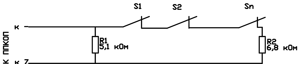
Рисунок 7 - Формирование шлейфа с двумя оконечными резисторами из нормально замкнутых датчиков
