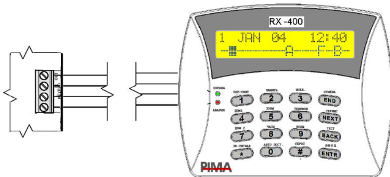
Рисунок 16 - Подключение клавиатур
