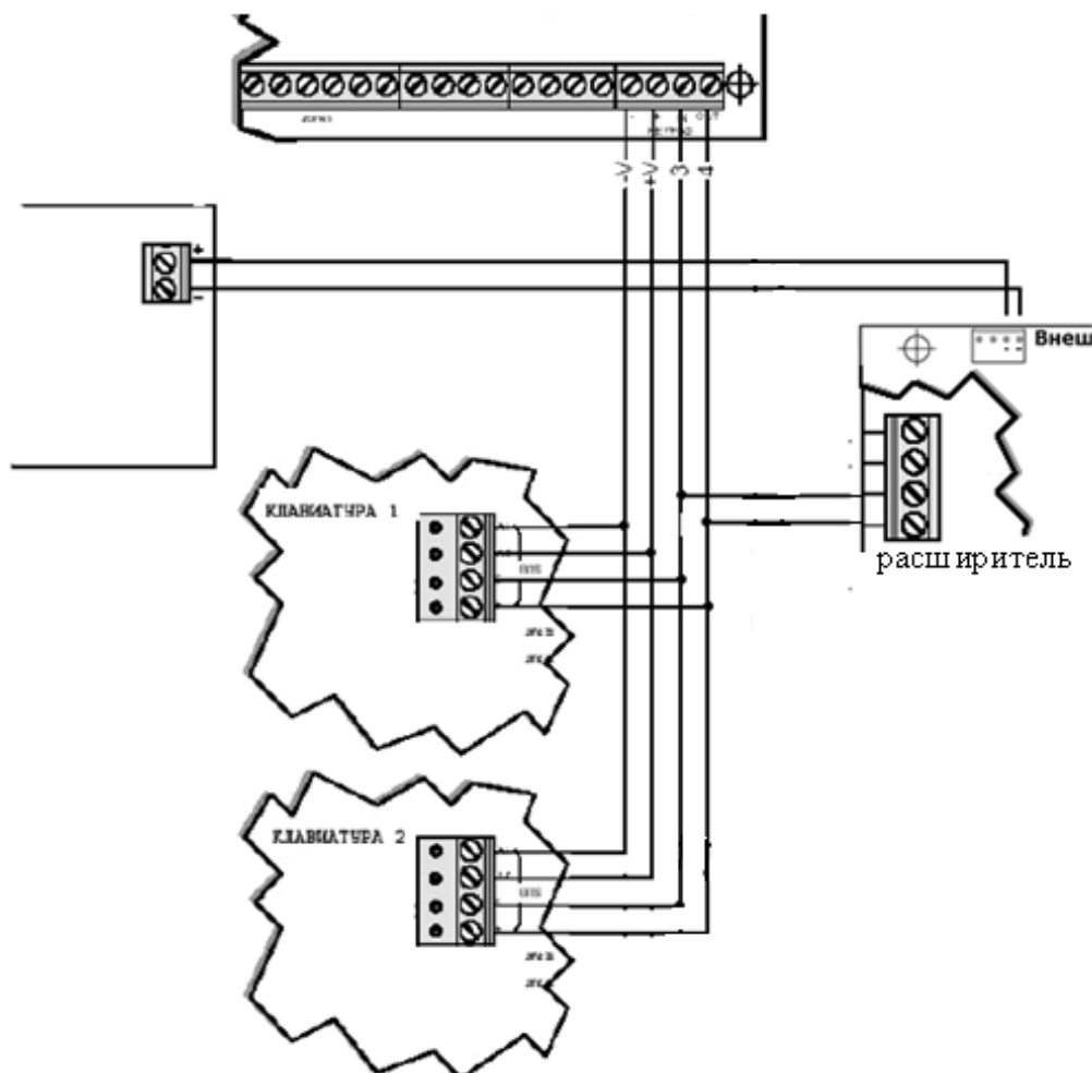
Рисунок 23 - Подключение расширителей и клавиатур с дополнительным источником питания, подключенным к внешнему разъему
