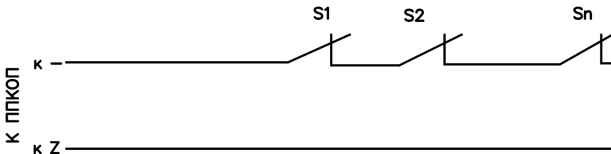
Рисунок 3 - Формирование шлейфа без оконечного резистора из нормально разомкнутых датчиков
