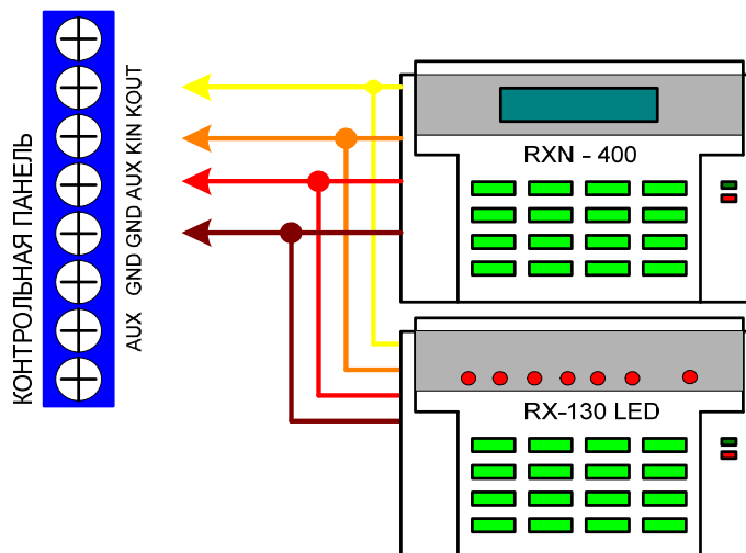
Рисунок 8 –Схема подключение различных типов клавиатур и устройств ввода кодов.
