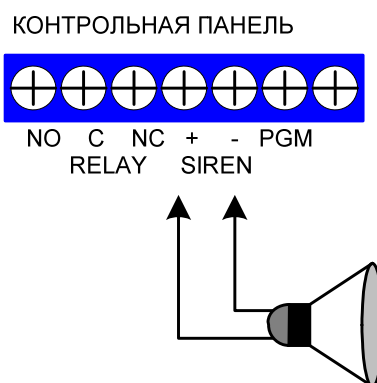
Рисунок 6 –Схема для подключения сирены.
