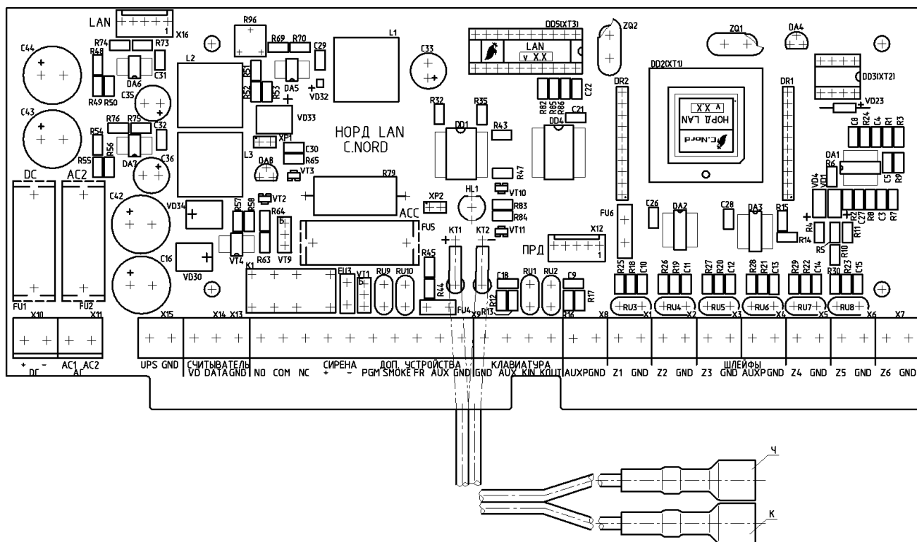
Рисунок 1 – Общий вид базовой платы прибора HOPD LAN
