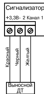
Рисунок 3 – Схема подключения выносной ДТ к сигнализатору
